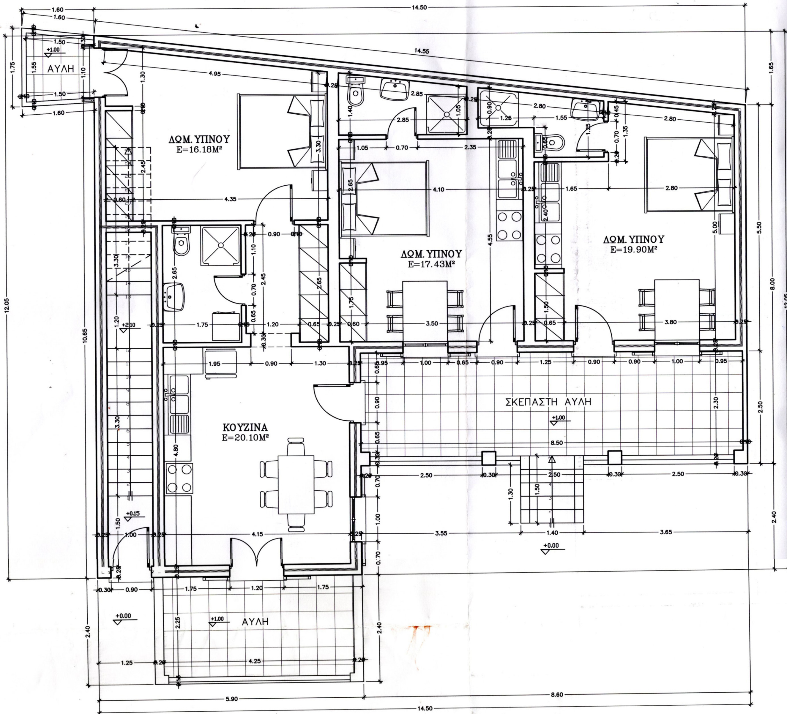
ΙΣΟΓΕΙΟ/GROUND FLOOR
